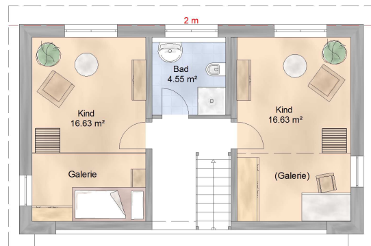
Erdgeschoss - Obergeschoss WFL: ca. 74 m 2
