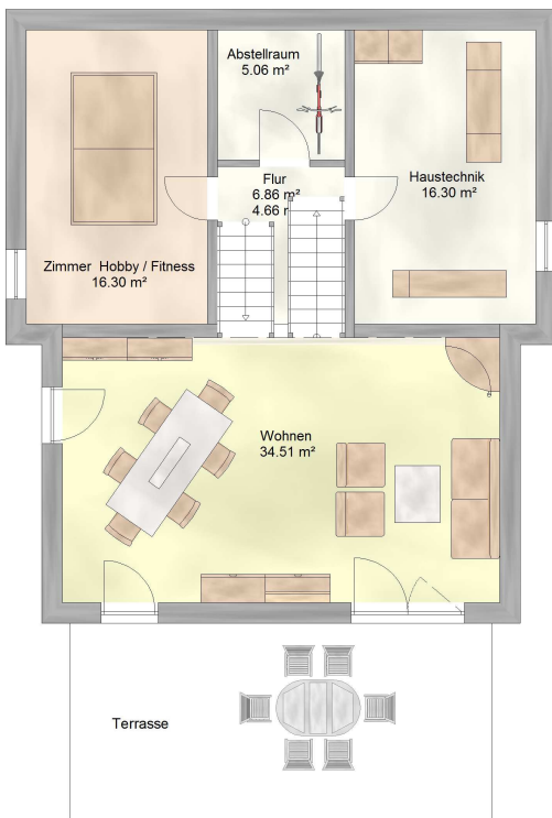
Kellergeschoss - Gartengeschoss WFL: ca. 77 m 2
