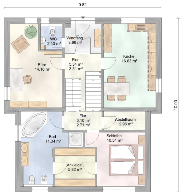
Erdgeschoss - Obergeschoss WFL: ca. 74 m 2
